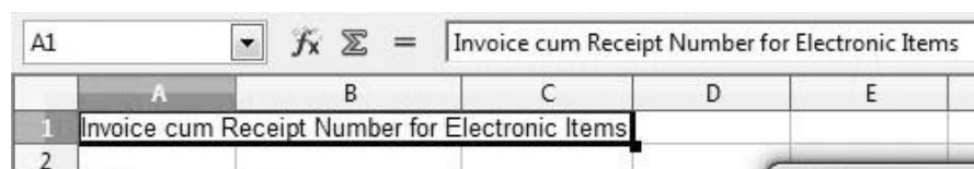
Fig. 9.25: Long text
