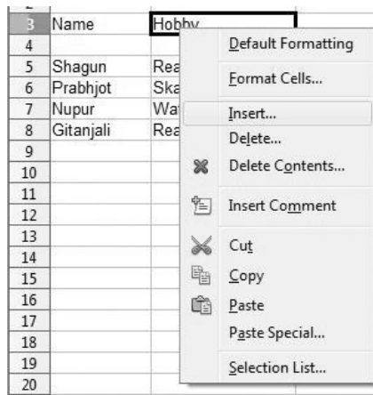
Fig. 9.15: Insert option
